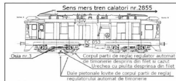
Figura nr.2 Schița loviturii dalelor pietonale de corpul părții de reglaj al regulatorului automat de timonerie al locomotivei EC 053.
